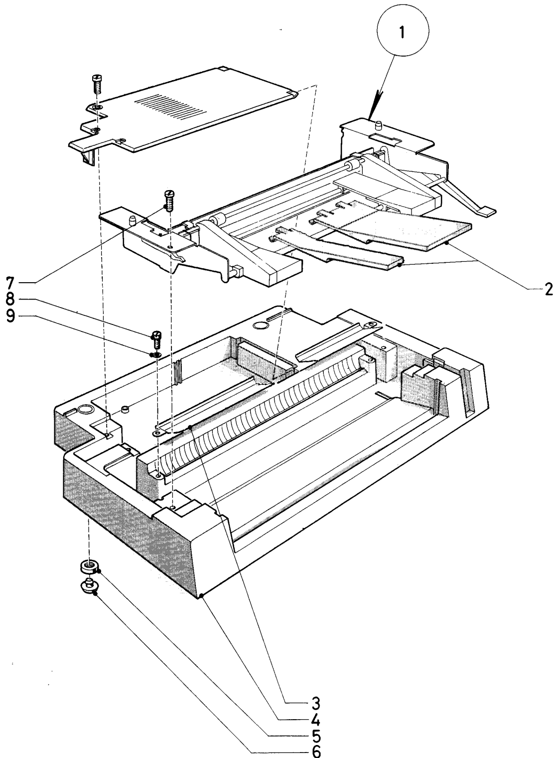
Figura 9-15 Assieme Caricatore Automatico di Moduli Doppio Cassetto Figure 9-15 Dual Bin Automatic Sheet Feeder Assembly
