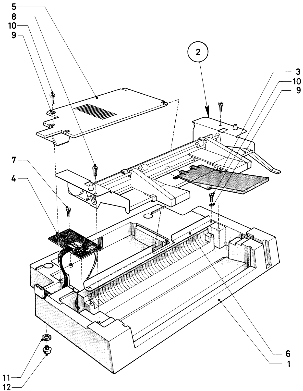
Figura 9-13 Assieme Caricatore Automatico di Moduli Cassetto Singolo Figure 9-13 Single Bin Automatic Sheet Feeder Assembly
