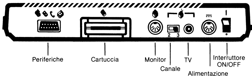
Connettore periferiche
